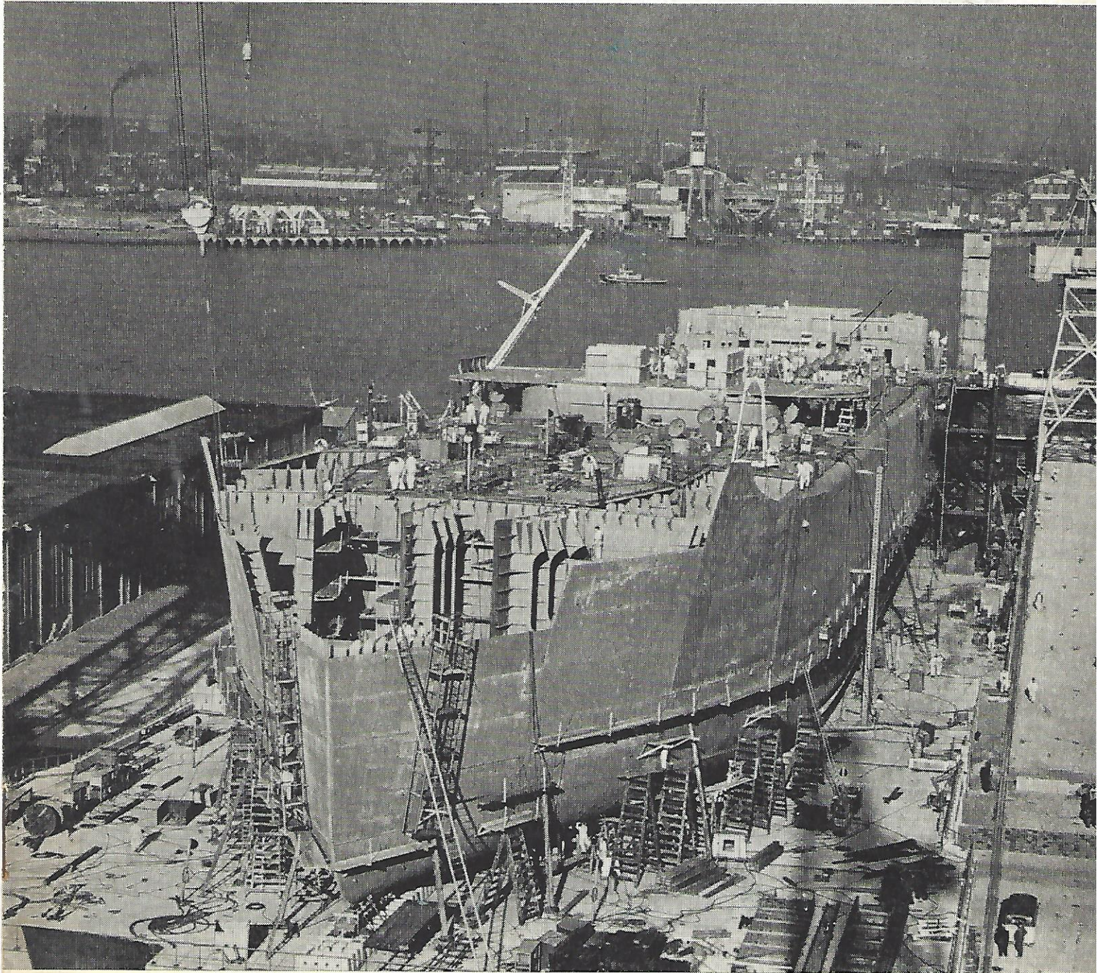
ONS NIEUWE VLAGGESCHIP - S.S. „ONDINA” - IN AANBOUW
